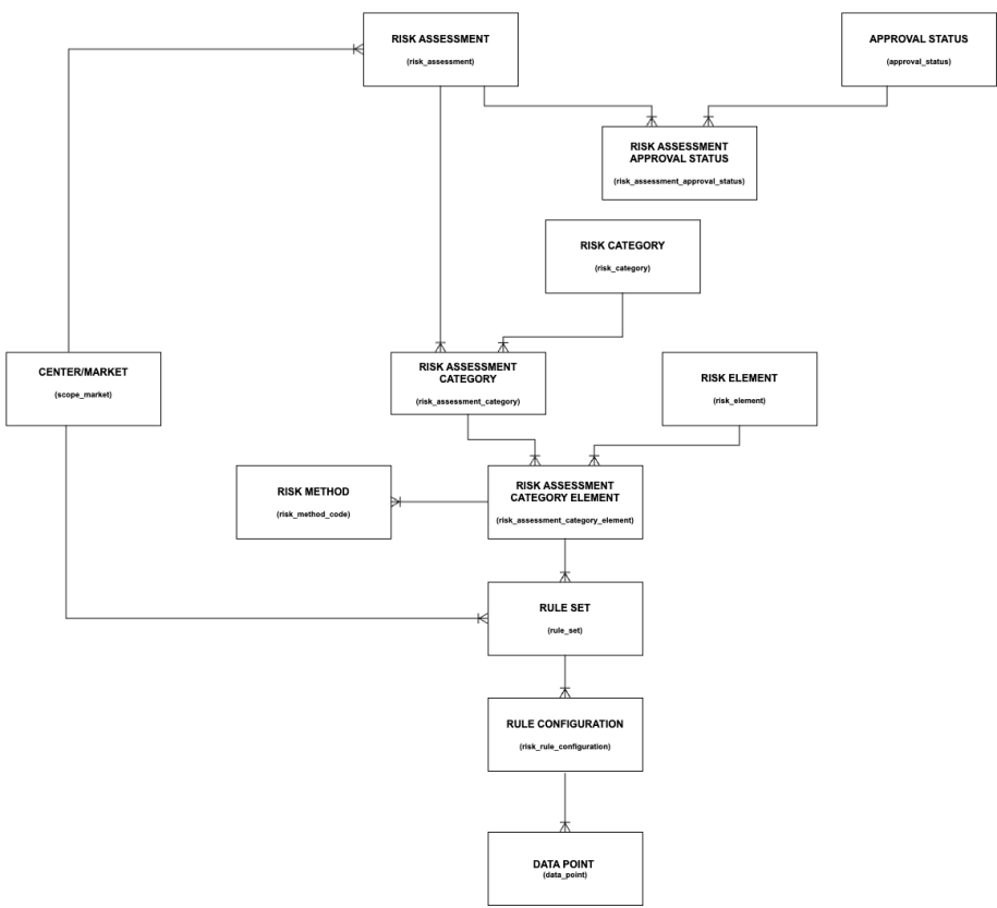
ER Diagram
